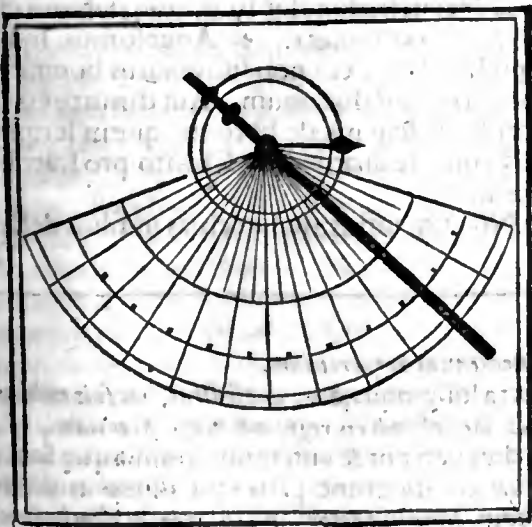
Figura secundum primam opinionem in qua duæ lineæ faciunt vnam horam.
