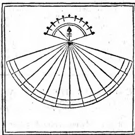
Figura secundum secundam opinionem in qua quælibet linea facit vnam horam.
